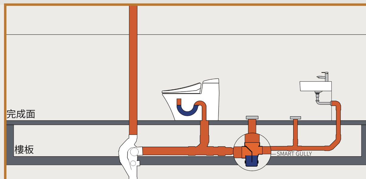
▲ 總存水彎+單管蘇維托系統
