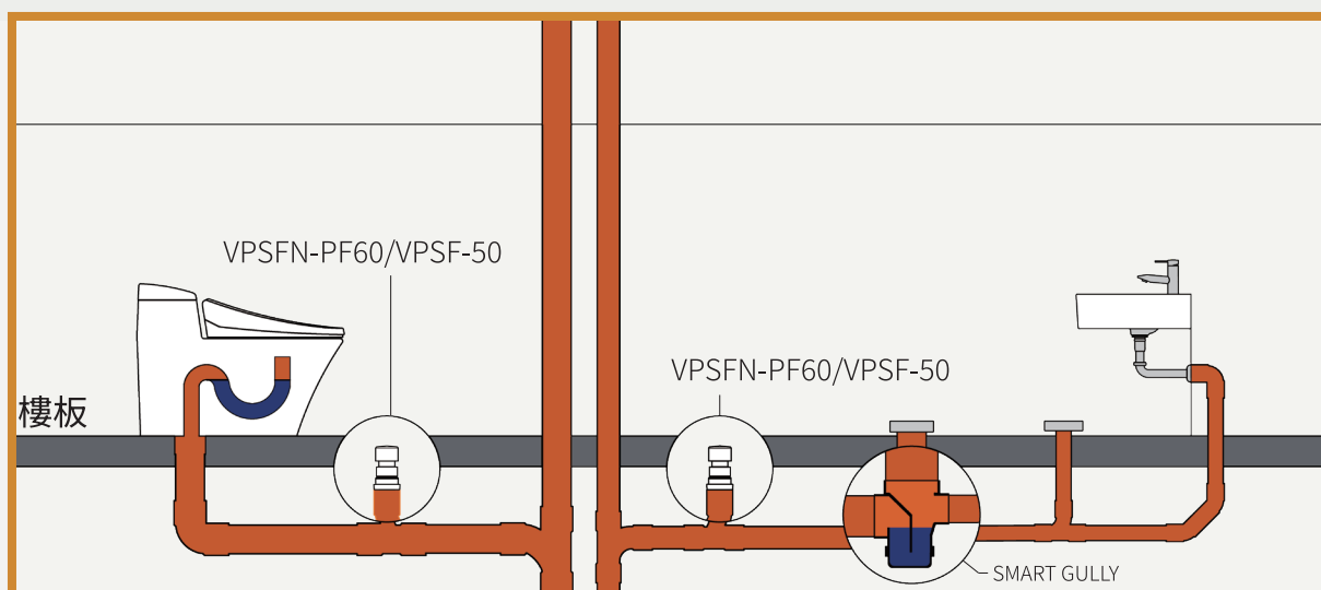
▲ 總存水彎+吸氣閥系統
