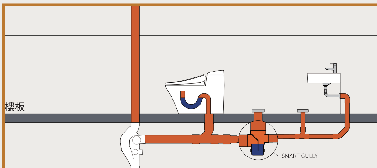
▲ 總存水彎+單管蘇維托系統
