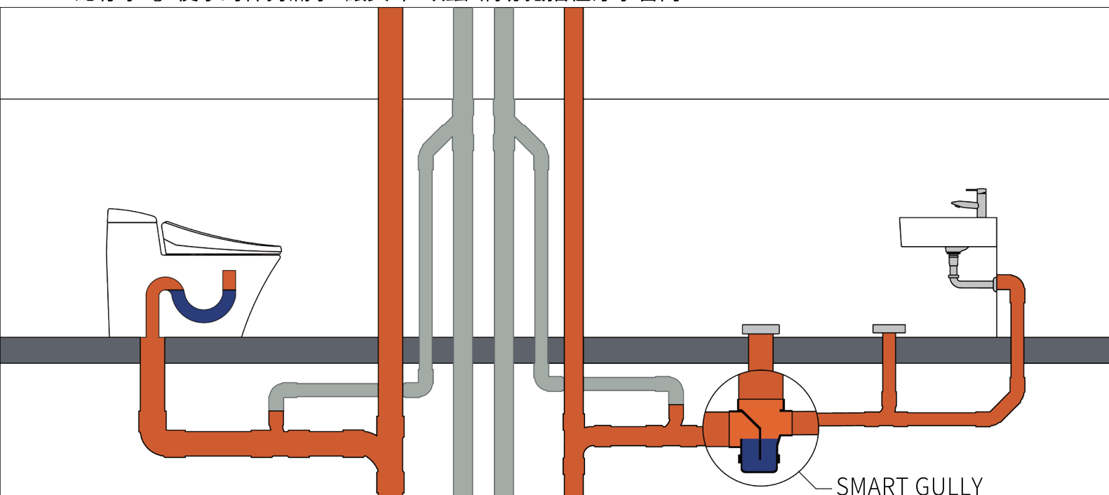
▲ 總存水彎系統工法示意圖
