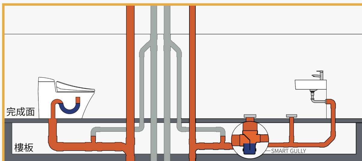
▲ 總存水彎+傳統透氣管系統
